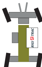
Verzögerte Lenkung (Patentiert)
